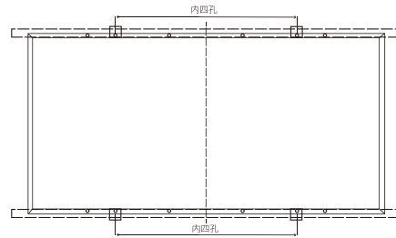
Installation par quatre trous intérieurs
