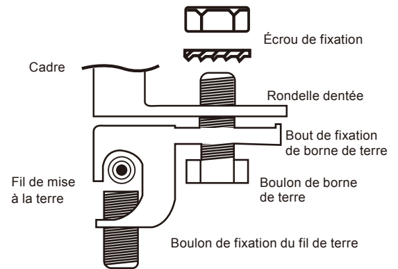
Figure 12 Méthode d'Installation
