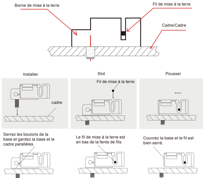
Figure 11 Installation de la borne de mise à la terre Remarque: TYCO. 1954381-1 (recommandé) est utilisé dans les figures ci-dessus.
