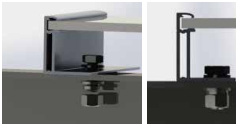
Figure 4 Méthode d'installation
