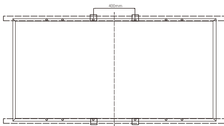
Installation à l'espace des trous de 400mm (La distance entre le côté C du cadre et le support est supérieure à 30 mm)
